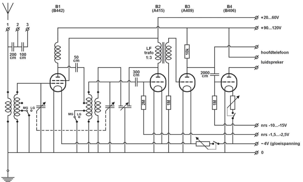
Schema van 4-lamps Venophon accutoestel, vastgesteld door Ries Kruidenier, hertekend door Gerard Jongbloed.
