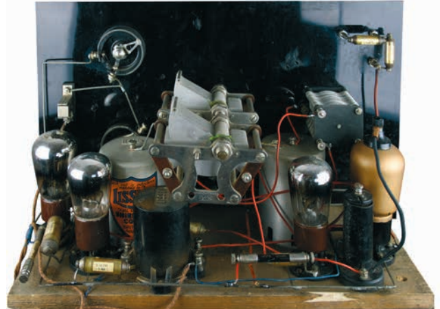
Chassis van de in 1943 in Hennaarderadeel ingeleverde Venophon-radio, thans in collectie van Ries Kruidenier.
